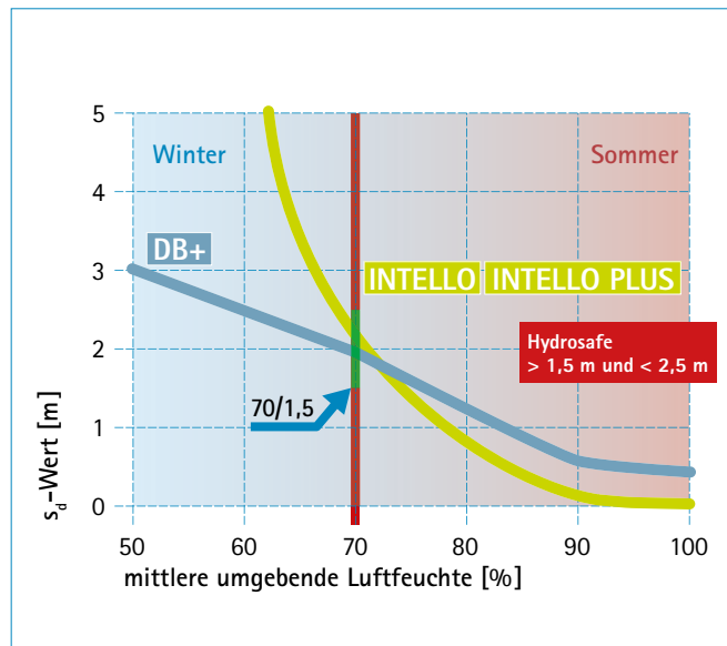
Abb. 6: Ein s_d -Wert zwischen 1,5 und 2,5 m bei 70 % rel. Luftfeucht sorgt nach DIN 68800-2 für sichere Bauteile während der Bauphase und der späteren Nutzung.
